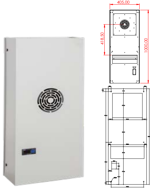
DİKİLİ TİP YAN KAPAK MONTAJ DIŞ ORTAM KLİMASI BOYALI KASA A SINIFI EKİPMAN
